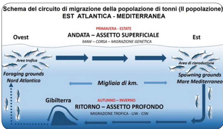
Fig. 6 – Schema esemplificativo del circuito di migrazione riguardante la II popolazione.
