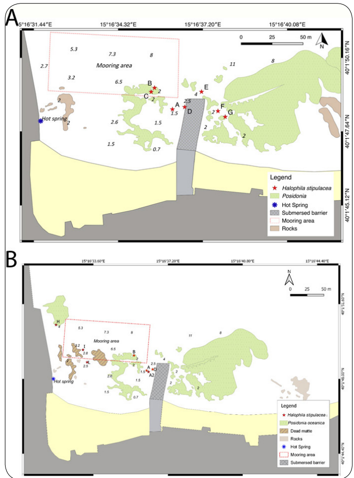
Fig. 2 - Distribuzione georeferenziata di H. stipulacea nel porto di Palinuro. A) Rilievi di aprile 2018 relativi alla distribuzione osservata ad ottobre 2017 (da Gambi et al. , 2018); B) rilievi di ottobre 2018, a seguito della presenza della specie anche lungo il molo (macchie L, I, H) (da Di Genio et al. , 2021).
