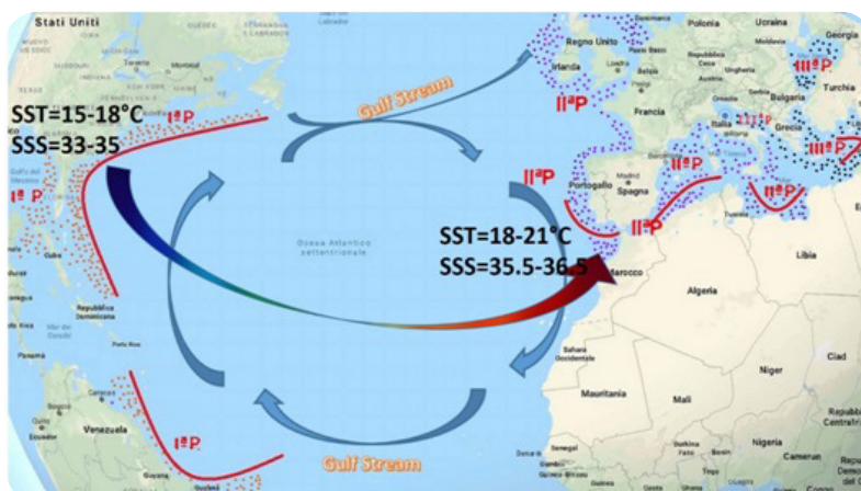
Fig. 3 – Gradiente di temperatura e salinità nel senso Ovest-Est.
