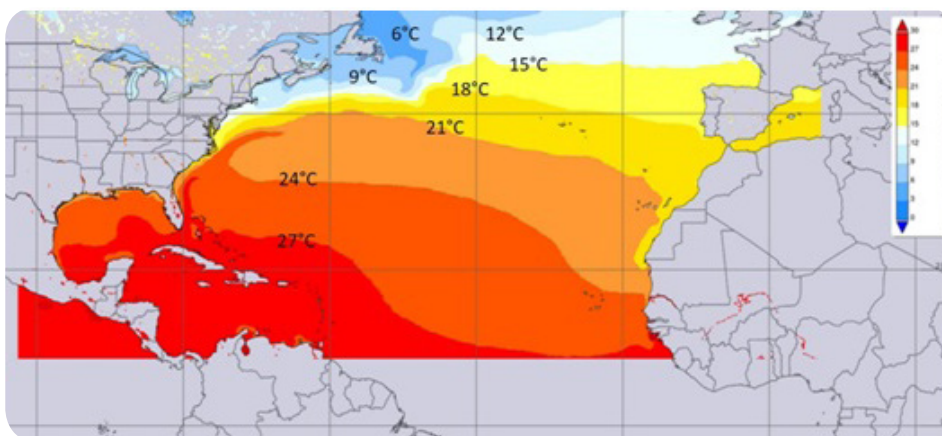
Fig. 8 – Mappa del gradiente di temperatura superficiale del mare prodotta con il sistema di dati online ( https://giovanngsfc.nasa.gov ) da Goddard Earth Sciences Data and Information Services Center (GES DISC), NASA.
