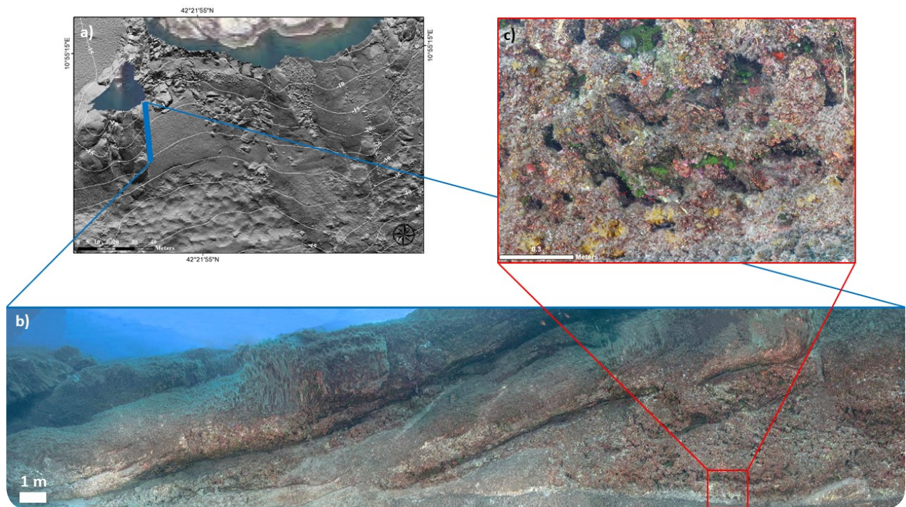
Fig. 10 - Esempio di ortofotomosaico effettuato lungo una parete verticale estesa alcune decine di metri ed evidenziata in blu nella mappa in alto a sinistra (a). Il fotomosaico (b) consiste nel generare un'ortofoto ottenuta mediante l'unione di numerose immagini con tecniche di image stitching. Le immagini di estese porzioni di fondale mantengono un elevato dettaglio a scala centimetrica (c) (da Casoli et al. , 2021)
